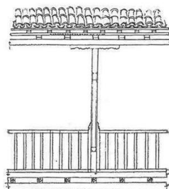
KORNIZA E STREHES
