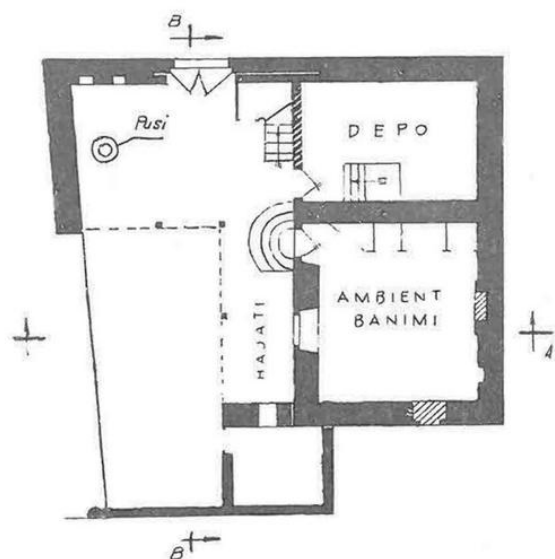
PLANIMETRIA E KATIT II
