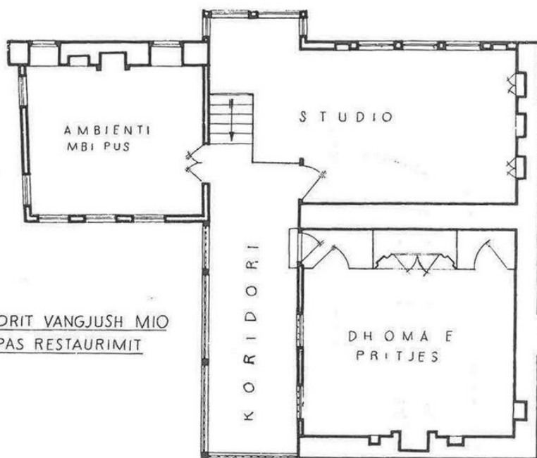
PLANIMETRIA E KATIT I
