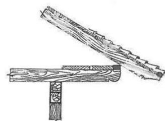
STREHA E ÇARDAKUT
