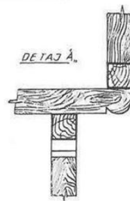
KORNIZA E STREHES
