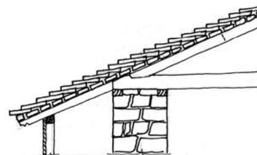
Prerje 1-1
