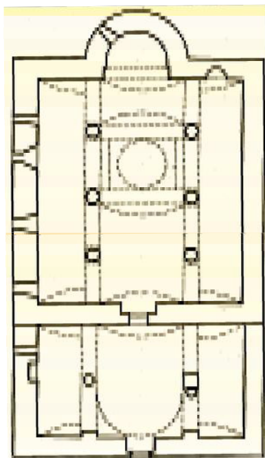
Κάτοψη του ναού.
