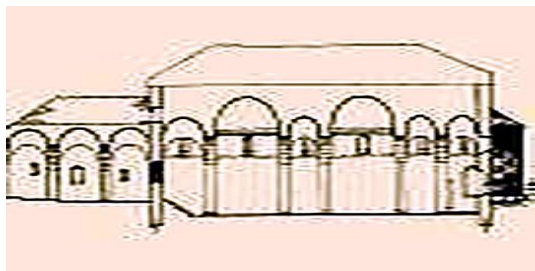
Prerja gjatësore.
