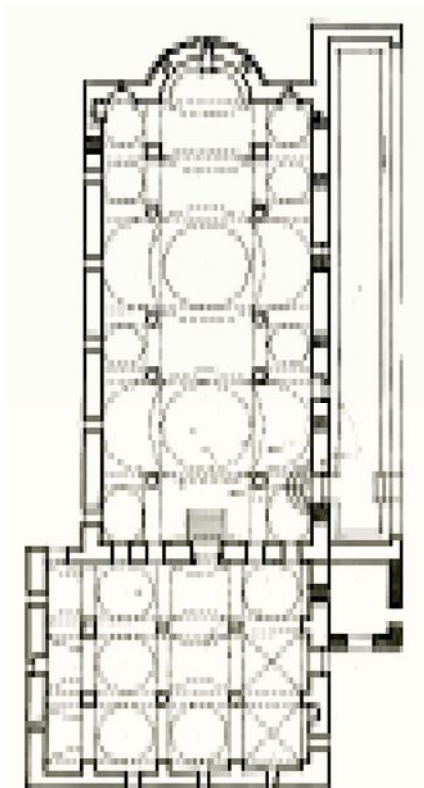
Planimetria e kishës së Taksiarkëve.
