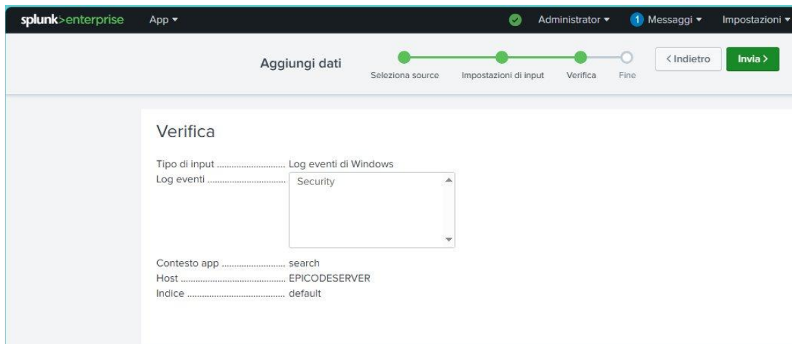
Fig. 2 - Riepilogo della configurazione prima dell'invio: Log eventi Windows, canale Security, host EPICODESERVER
