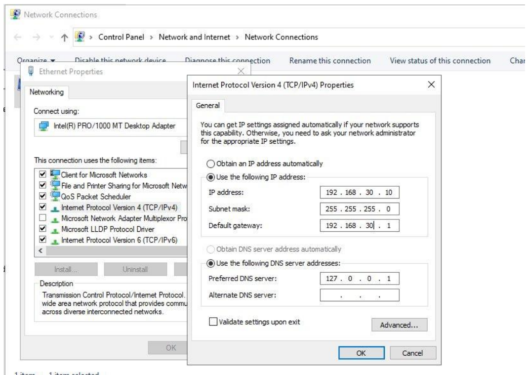
Configurazione IPv4 della scheda di rete del server
