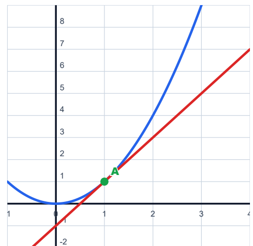
La tangente (rouge) à la courbe y = x^2 au point A(1 ; 1) : sa pente est f'(1) = 2 .
