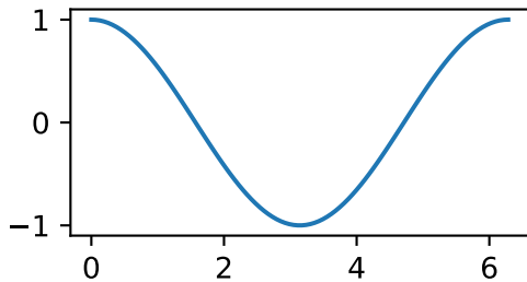
\cos(x)
