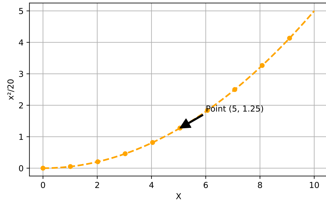
Quadratic function
