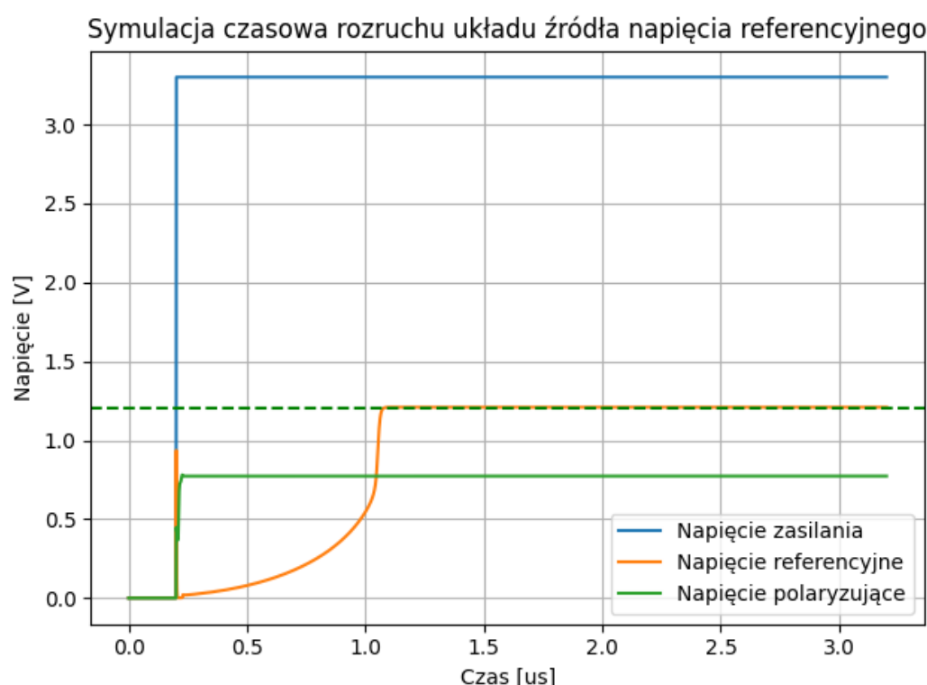
Rys 8.4: Symulacja czasowa rezystorowego układu źródła napięcia odniesienia. Linia przerywana wskazuje pożądaną poziom generowanego napięcia wyjściowego (1,2V). Symulacja wykonana z zerowymi warunkami początkowymi. Symulacja wykonana po ekstrakcji parametrów pasożytniczych.
