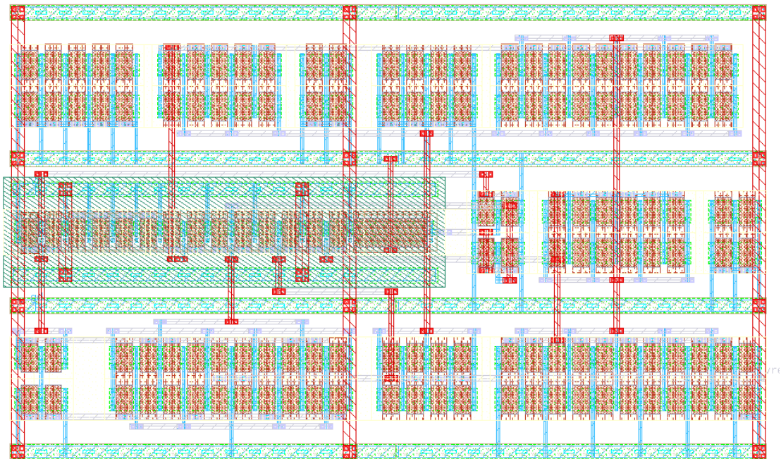
Rys 7.2: Topografia zaprojektowanego bezrezystorowego układu źródła napięcia odniesienia. Wymiary topografii: 40,83 \times 24,56 \mu\text{m} .
