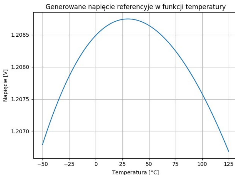
Rys 8.3: Charakterystyka generowanego napięcia odniesienia w funkcji temperatury. Symulacja wykonana po ekstrakcji parametrów pasożytniczych.
