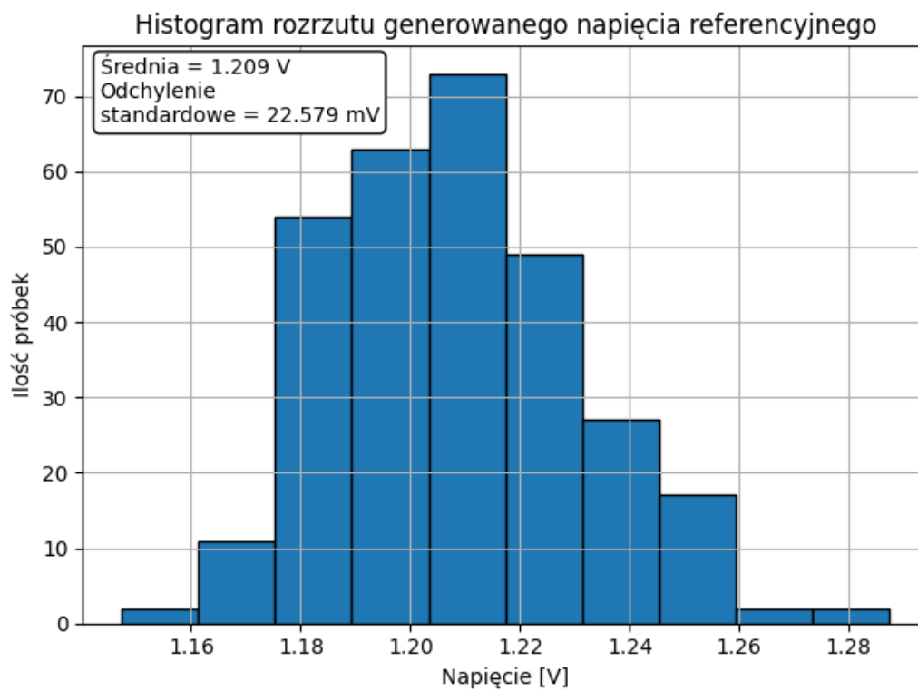
Rys 8.5: Histogram rozrzutu generowanego napięcia referencyjnego. Analiza Monte Carlo dla 300 próbek.
