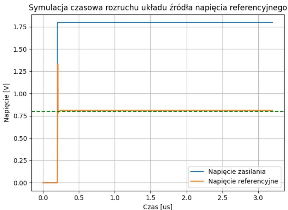
Rys 8.7: Symulacja czasowa bezrezystorowego układu źródła napięcia odniesienia. Linia przerywana wskazuje pożądaną poziom generowanego napięcia wyjściowego (0,8V). Symulacja wykonana z zerowymi warunkami początkowymi. Symulacja wykonana po ekstrakcji parametrów pasożytniczych.
