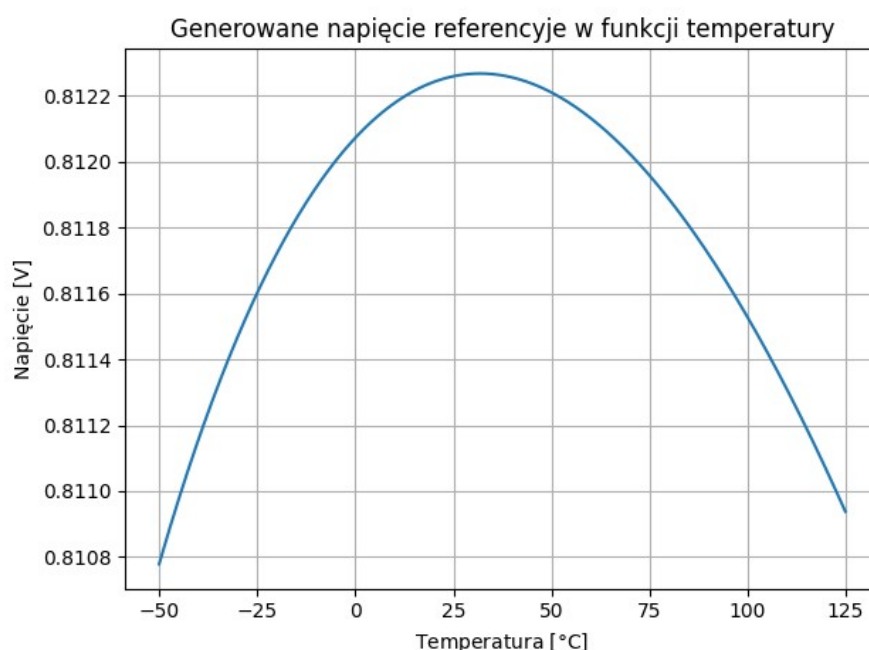
Rys 8.6: Charakterystyka napięcia odniesienia generowanego przez układ bezrezystorowy w funkcji temperatury. Symulacja wykonana po ekstrakcji parametrów pasywnych.
