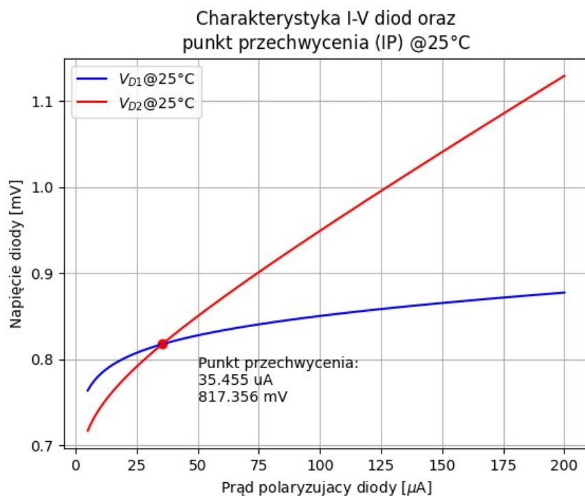
Rys 8.2: Charakterystyki przedstawiający punkt przechwycenia dla całkowitego prądu polaryzującego (suma prądu diody oraz prąd rezystora CTAT) 100 \mu\text{A} .
