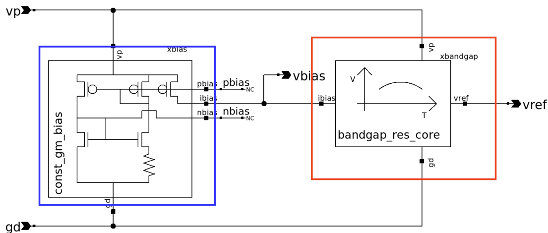
Rys 6.4: Schemat finalnego projektu układu rezystorowego. Na rysunku zaznaczono: rdzeń układu źródła napięcia odniesienia (czerwona ramka) oraz układ polaryzujący (niebieska ramka).
