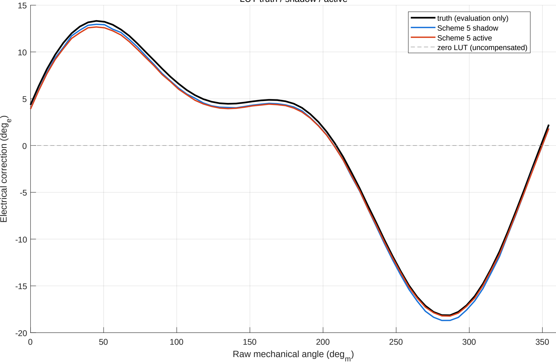
LUT truth / shadow / active
