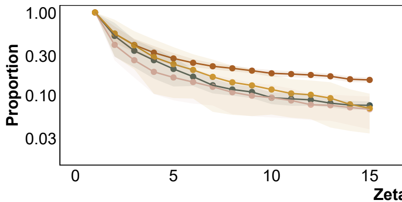
18S
