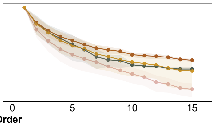
COI
