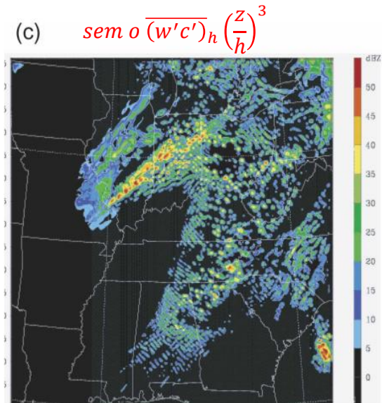
maximum (dBZ) at (a) 1800 UTC (d) 10 Nov 2002
