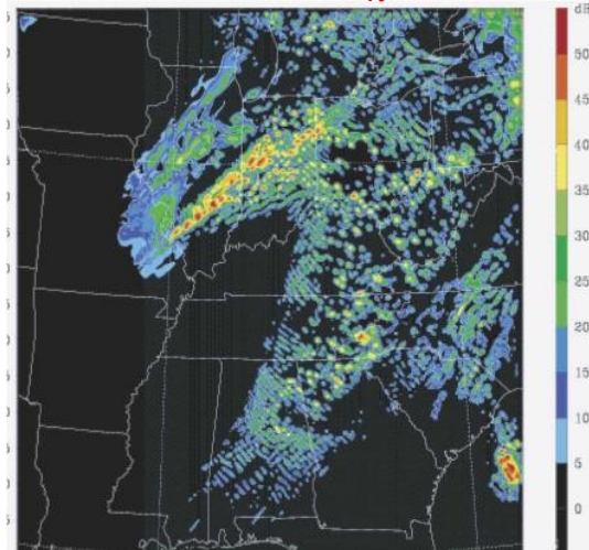
maximum (dBZ) at (a) 1800 UTC (d) 10 Nov 2002
