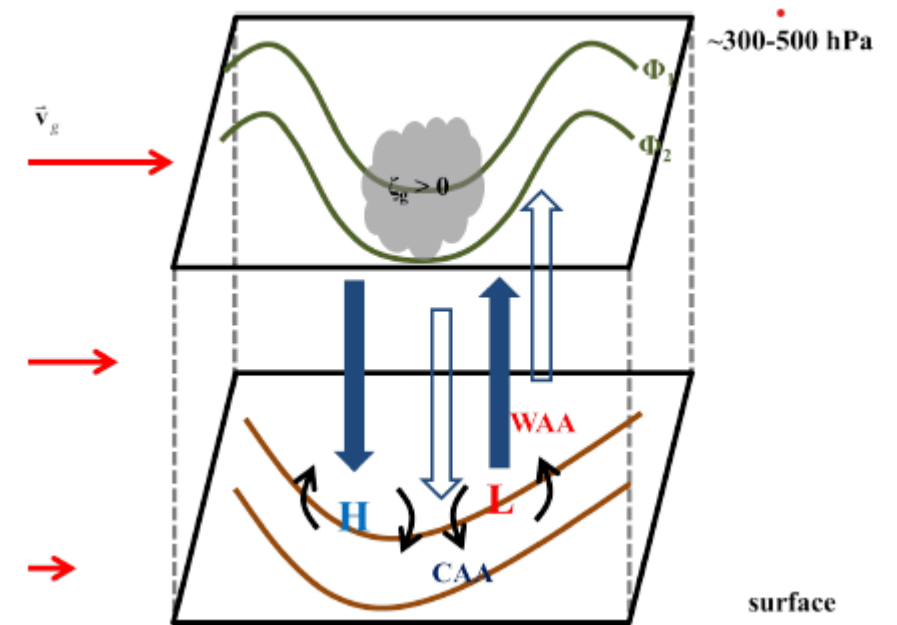
“Figura 4. Esquema idealizado do padrão da troposfera superior e inferior e os forçamentos associados à fase de desenvolvimento maduro de um ciclone de superfície em escala sinótica.”
