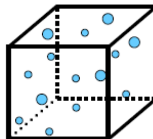
RAIN
