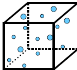
RAIN
