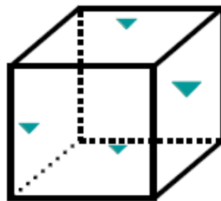
GRAUPEL
