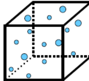
RAIN
