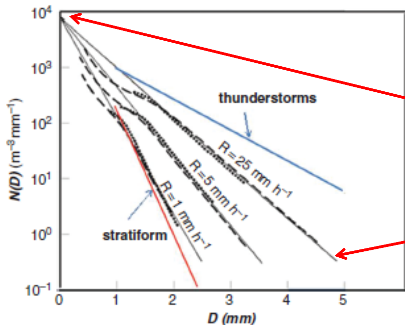
Figura 2.3.15 Distribuições médias de tamanho de chuva.
