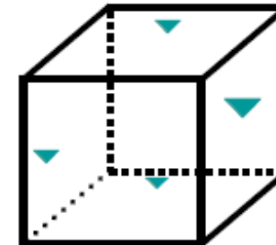
GRAUPEL
