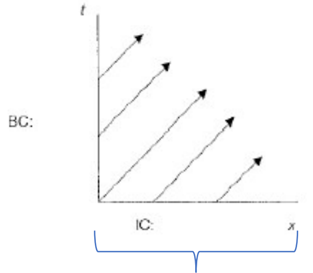
(a) velocidade positiva
