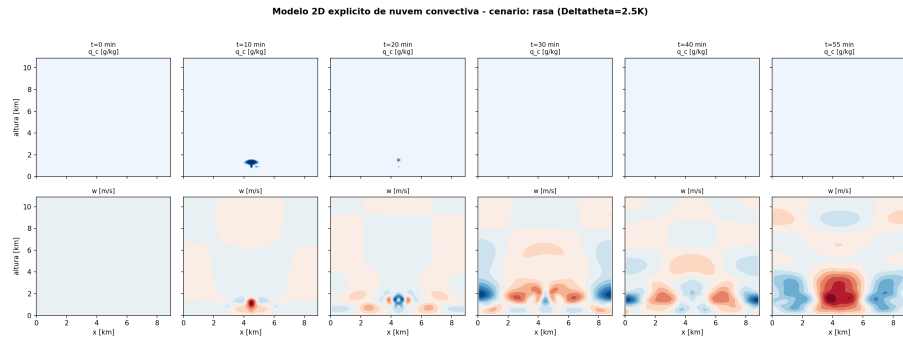
Figura 4.4 - Evolução da nuvem 2D com bolha térmica fraca (regime raso).
