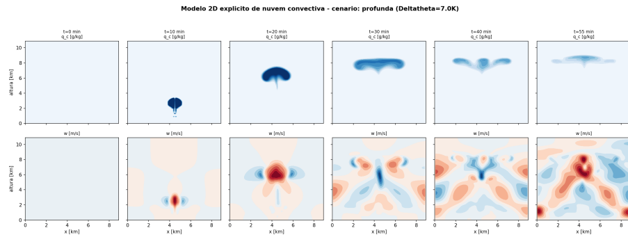
Figura 4.5 - Evolução da nuvem 2D com bolha térmica forte (regime profundo).
