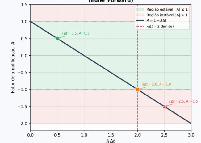
Diagrama de Estabilidade (Euler Forward)
