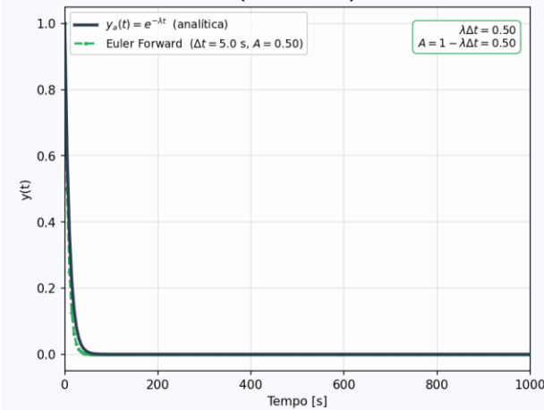
Solução Numérica vs Analítica (caso estável)
