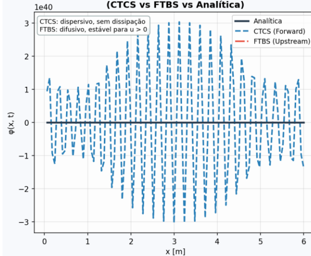
Comparação no passo tn = 20000 (CTCS vs FTBS vs Analítica)
