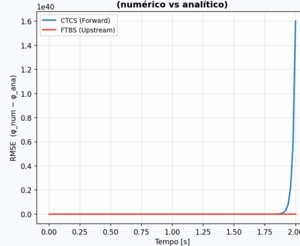
Erro RMS ao longo do tempo (numérico vs analítico)
