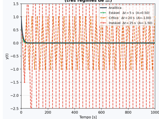
Comparação de Estabilidade (três regimes de \Delta t )
