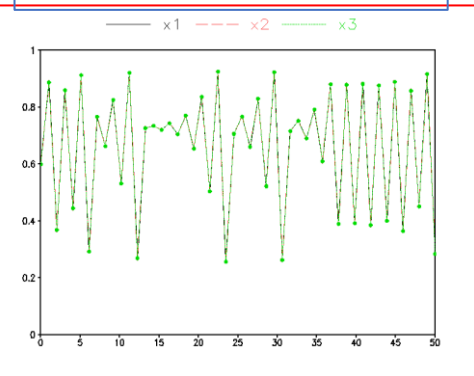
Diferença entre x_1 , x_2 e x_3 = 0
