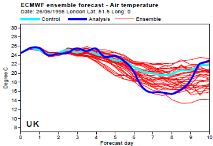
Figura 4. Previsões do ECMWF para a temperatura do ar em Londres iniciadas em:
