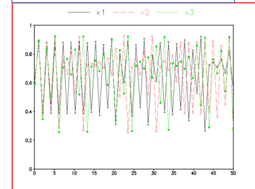
Diferença entre x_1 , x_2 e x_3 = 0.01
