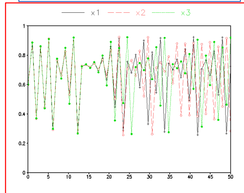
Diferença entre x_1 , x_2 e x_3 = 1e-5
