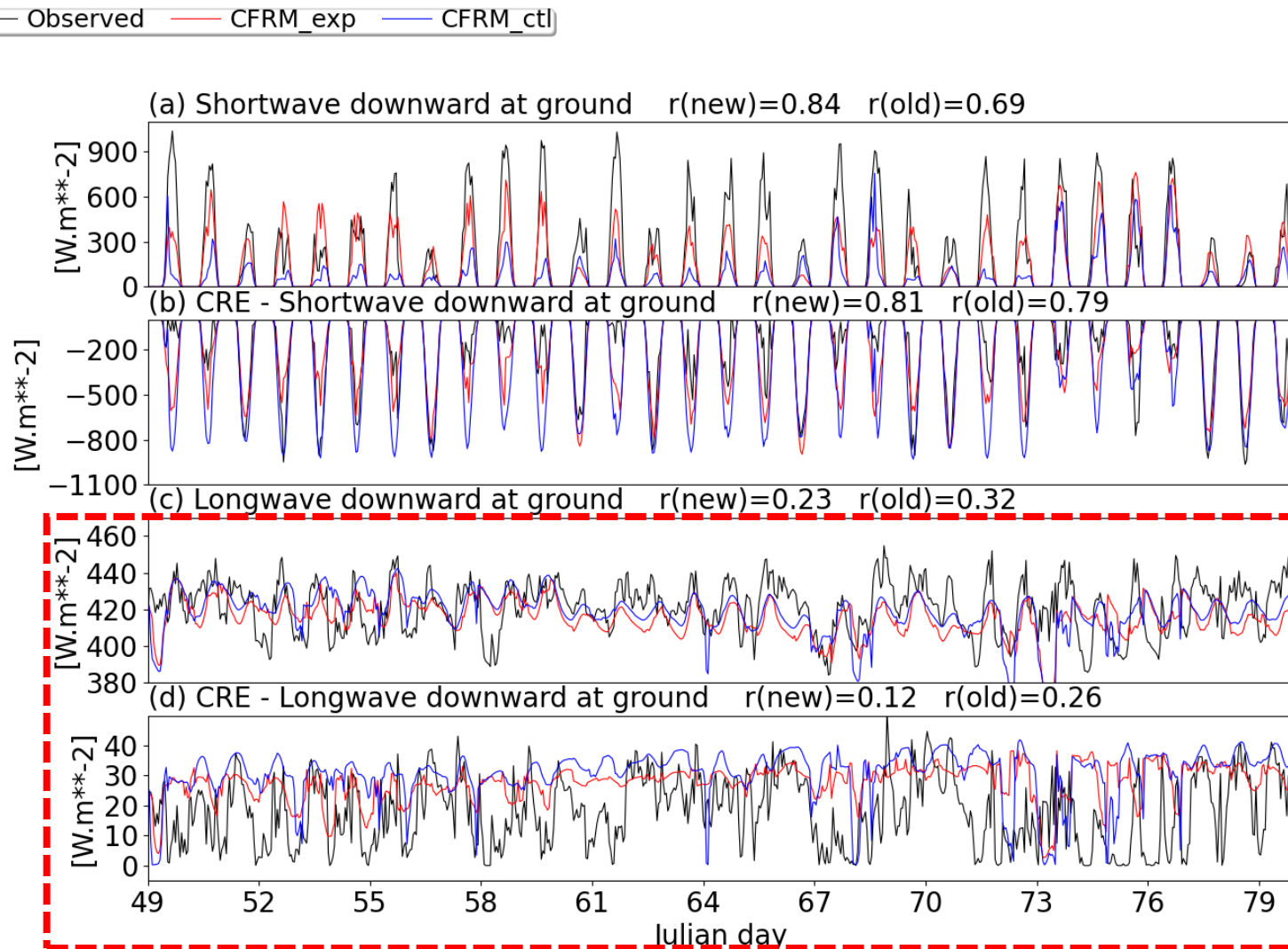
Figura 5.4 - Série temporal dos fluxos de radiação e efeito radiativo de nuvens (CRE) para o período da IOP1 do GoAmazon 2014/15. Simulações utilizando os dados do SAM como forçantes de larga escala.
