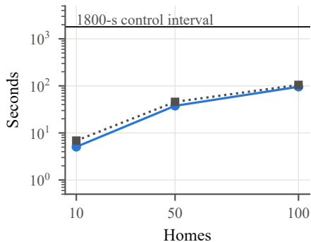
PJ-ADMM time per step
