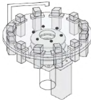
중공을 이용한 공정도 위치 결정 용도
