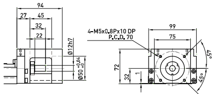
Motor connection flange F1
