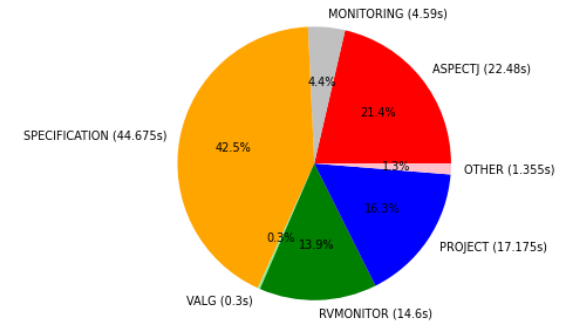
kiara (17.579s)
