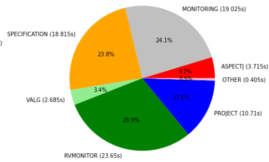
java.math.expression.parser (23.173s)
