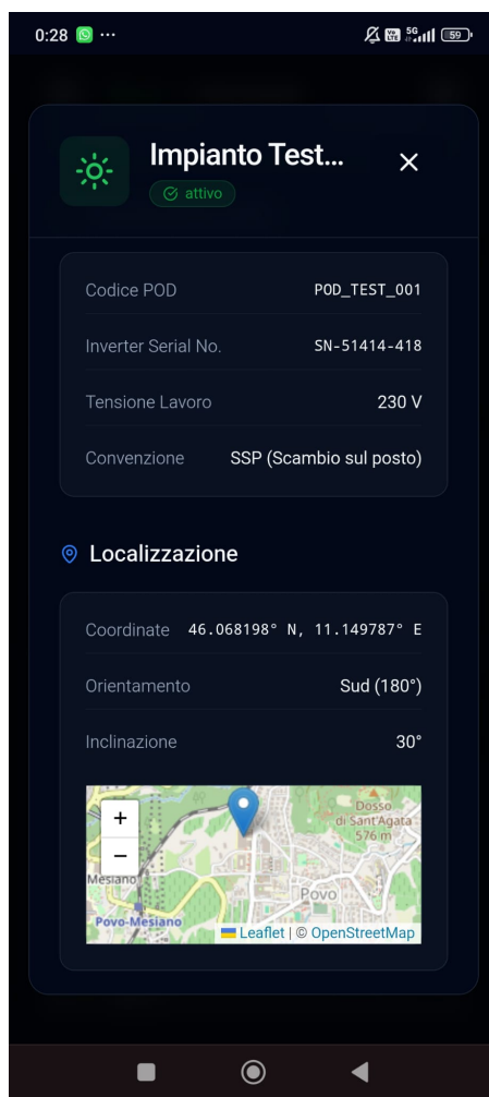
Figura 4: Gestione Impianti: Vista Desktop (sopra) con una visualizzazione tabellare per il riepilogo della potenza installata, dello stato operativo e Vista Dettaglio Mobile (sotto), con dettagli tecnici dell'impianto e integrazione mappa Leaflet per la posizione. Funzionalità di segnalazione guasti e manutenzioni sono accessibili in layout Desktop e Mobile tramite menù a tendina.
