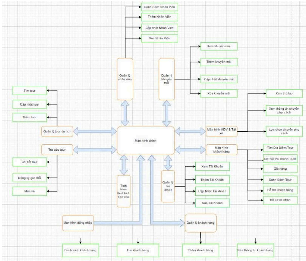
Hình 4-1. Danh sách các màn hình và sơ đồ chuyển đổi
