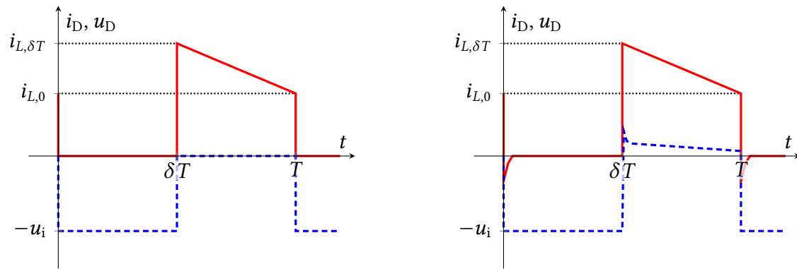
Abbildung 2.7: Spannungs- und Stromverlauf im Abwärtswandler. Links: Ideale Diode Rechts: Reale Diode.
