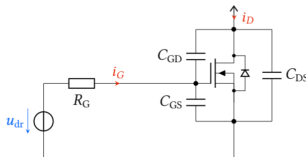
Abbildung 2.7: Interne parasitäre Kapazitäten eines MOSFETs.
