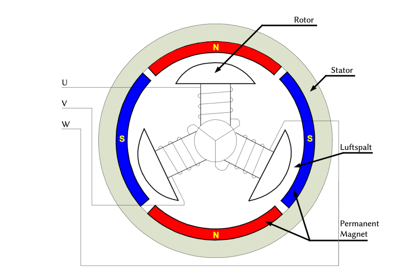
Abbildung 2.1: Querschnitt und prinzipieller Aufbau eines BLDC-Motors. Nach [1, Abb. 5b].
