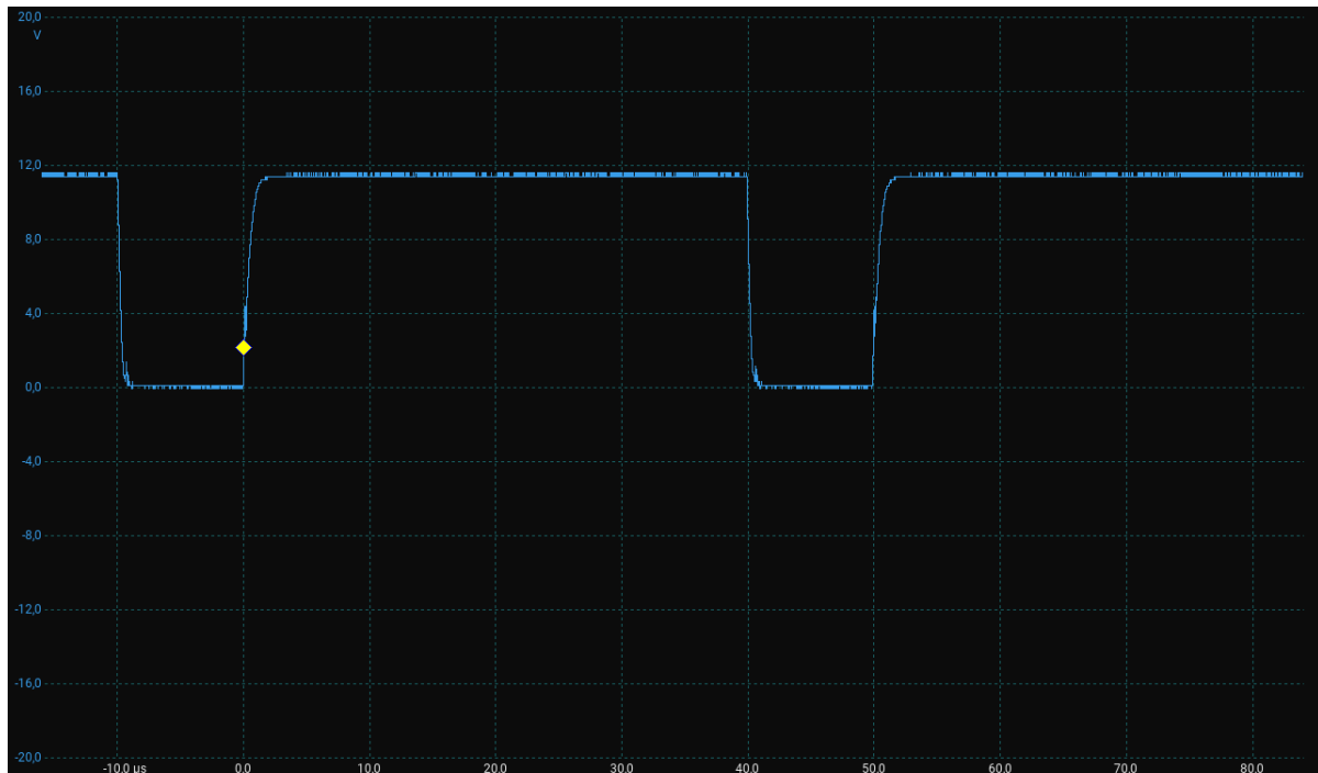
Abbildung A.5: Aktiver Sektor (PWM mit 20 kHz) mit Synchrongleichrichtung am LS-Gate. Zeitbasis: 10 \mu\text{s}/\text{div} .
