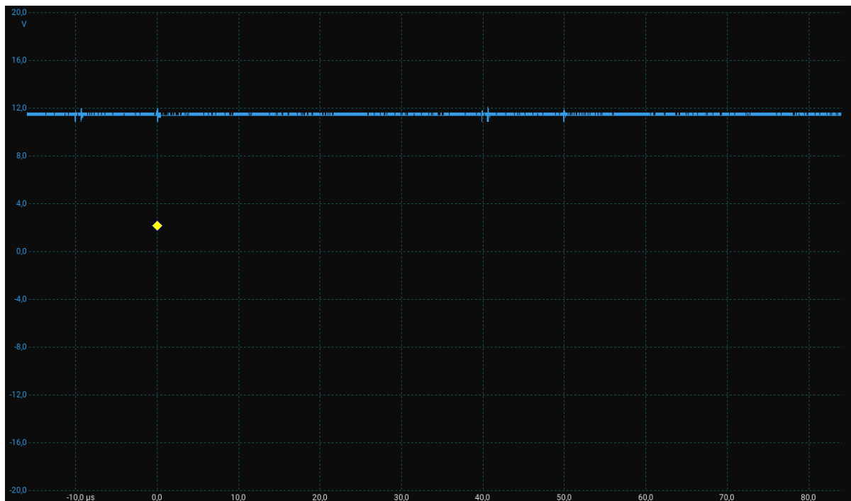
Abbildung A.6: Rückleiter-Betrieb mit statisch voll durchgesteuertem LS-Gate. Zeitbasis: 10 \mu\text{s}/\text{div} .
