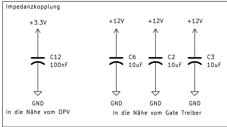
Abbildung 4.5: Hochfrequente Entkopplung der Logik- und Treiberspannungen.
