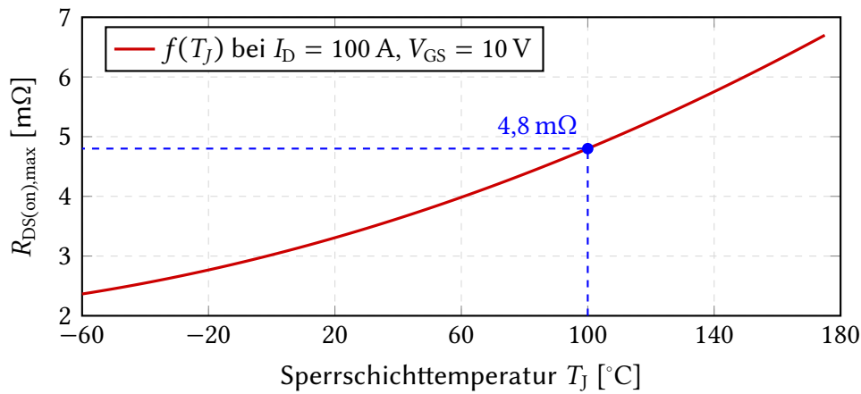
Abbildung 4.2: Temperaturabhängigkeit des maximalen Einschaltwiderstands. Grafisch ermittelter Arbeitspunkt bei 100^{\circ}C . Eigene Digitalisierung nach [6, Diagramm 9].
