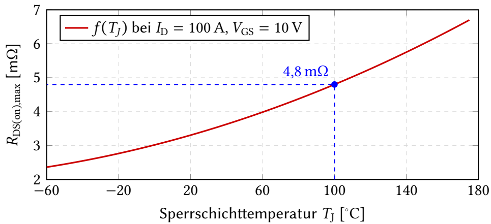
Abbildung 4.1: Temperaturabhängigkeit des maximalen Einschaltwiderstands. Digitalisiert nach [9, Diagramm 9].
