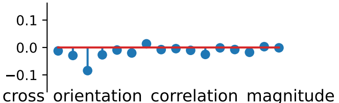
magnitude_std
