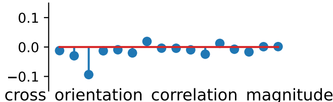
magnitude_std
