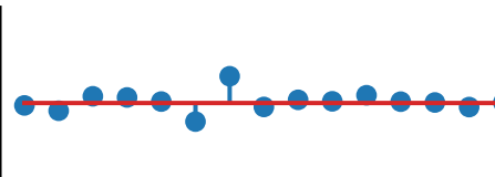
auto_correlation_magnitude
