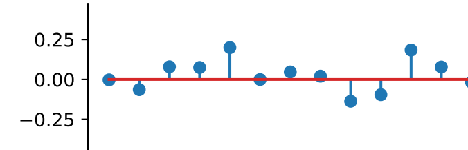
auto_correlation_magnitude
