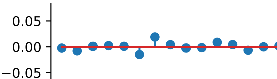
auto_correlation_magnitude
