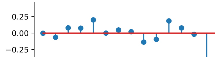
auto_correlation_magnitude
