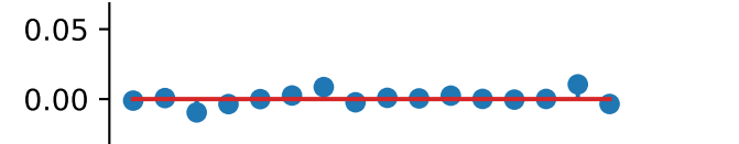
magnitude_std
