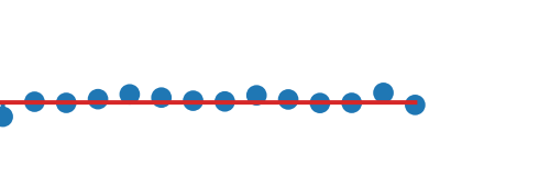
magnitude_std
