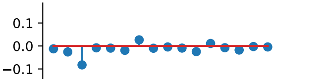
magnitude_std
