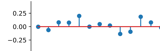
auto_correlation_magnitude
