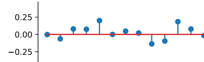
auto_correlation_magnitude
