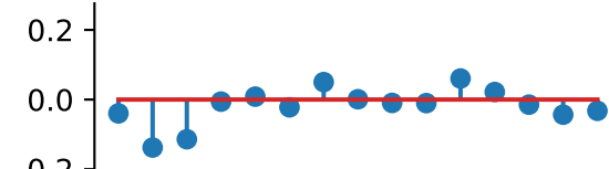
auto_correlation_magnitude
