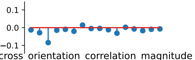
magnitude_std
