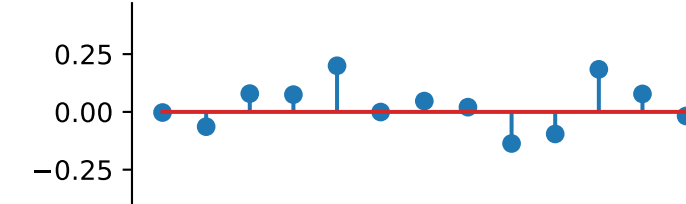
auto_correlation_magnitude
