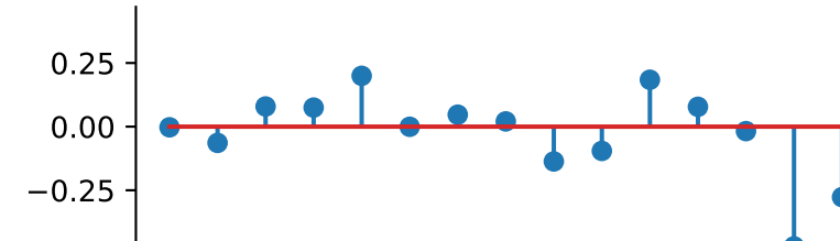
auto_correlation_magnitude
