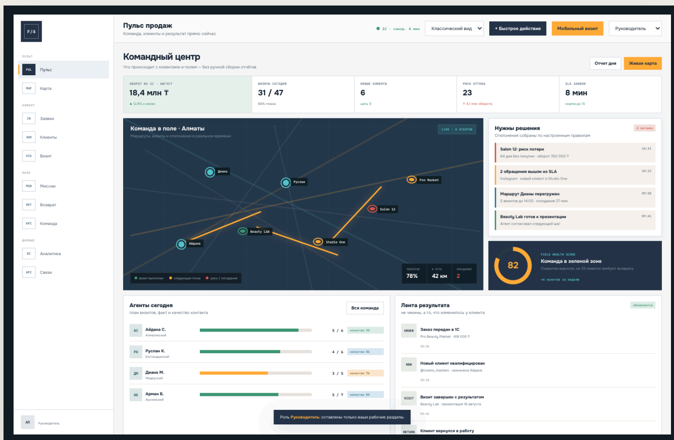
ЭКРАН 01 · Пульт продаж: команда в поле, сигналы и результат
